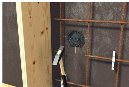
Přesné umístění díky integrovaným značkám na víku. Integrované upevnění hřebíky ve víku umožňuje snadnou montáž.
