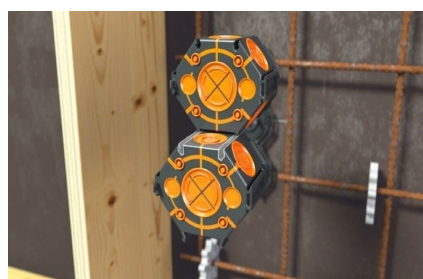
Spojovací technologie SCS - pevné spojení a snadné průběžné propojení vodičů.
