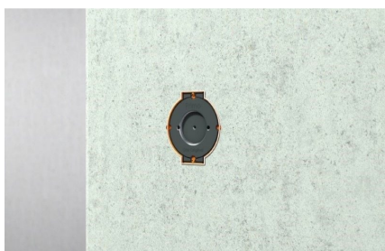
Montáž po betonáži: Těsnicí lem membrány je ideální pro pohledový beton.
