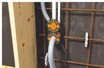
Kombinované zavedení kabelů a trubek M15-M32 bez použití nářadí. Membránová technologie zajišťuje dokonalou těsnost v betonu.
